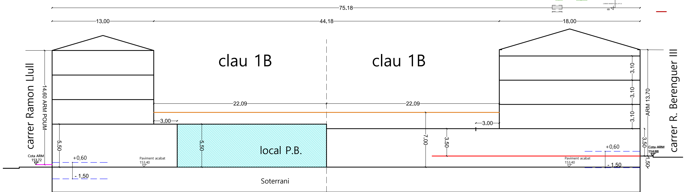
SECCIÓ B-B
