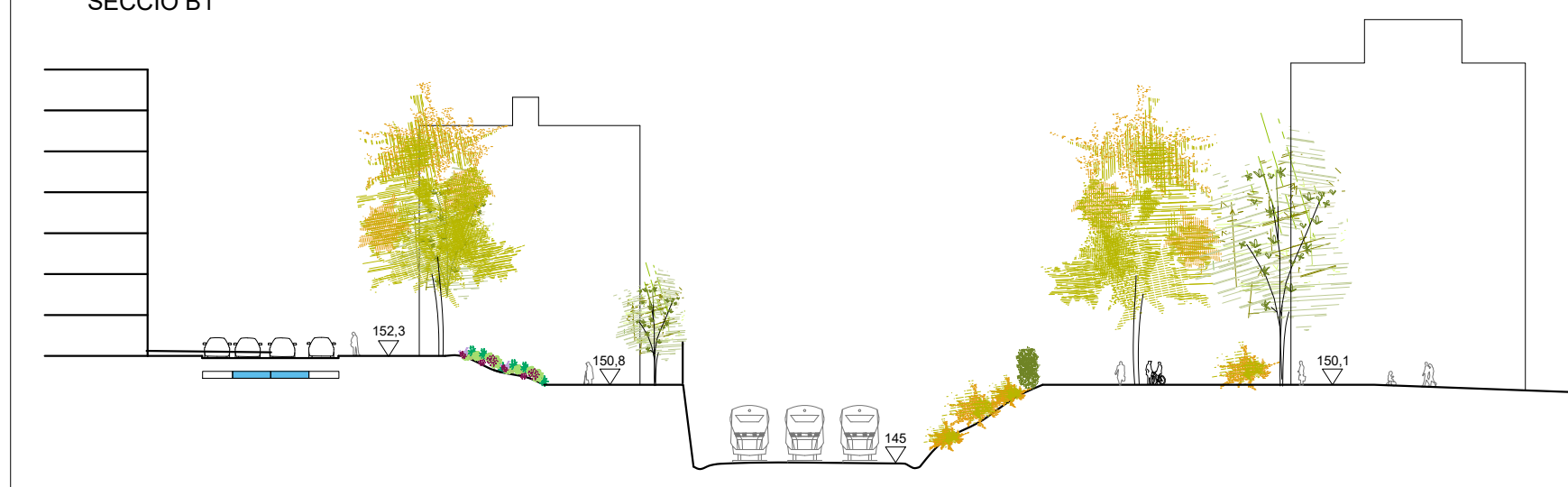
SECCIÓ B1
