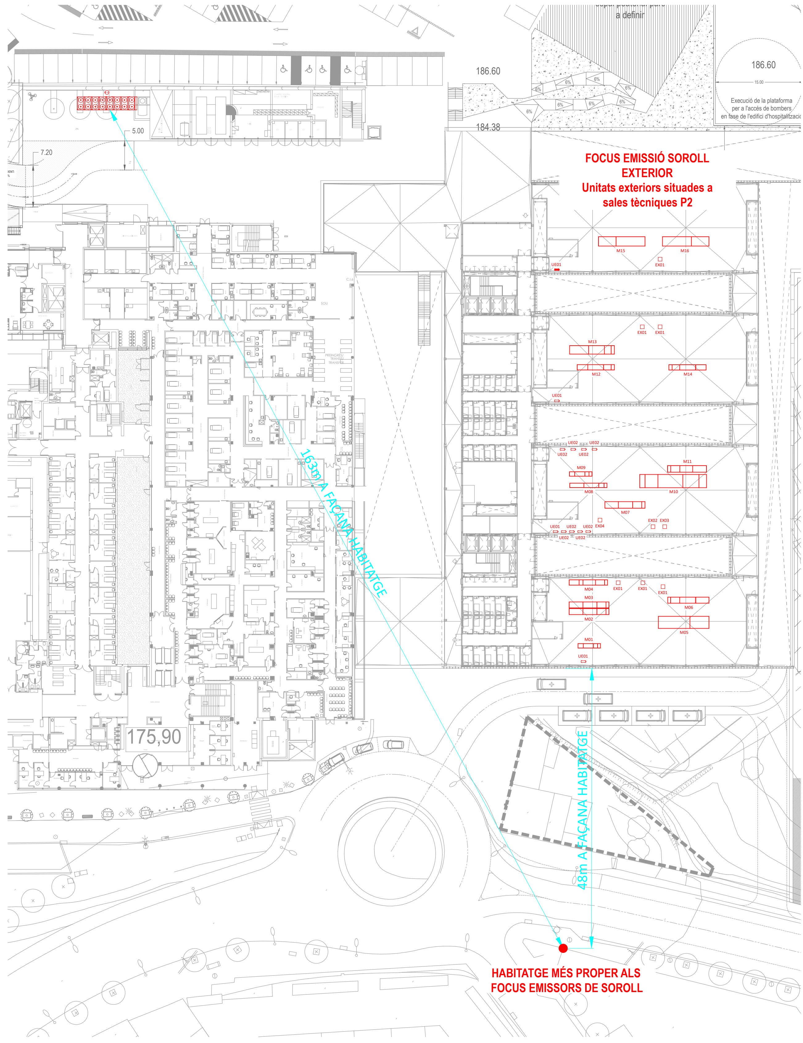
PLANTA SEGONA
