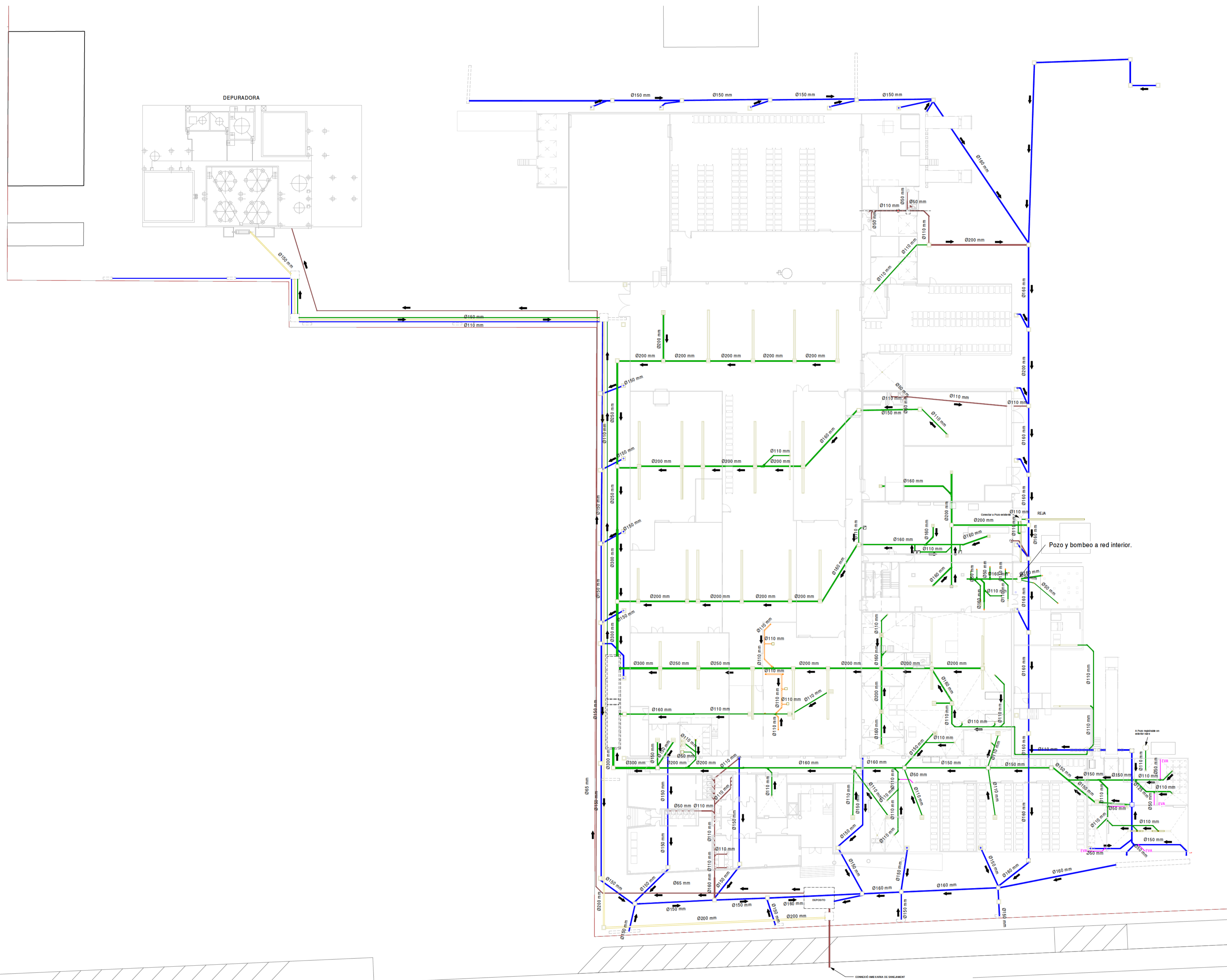
1 SANEAMIENTO GENERAL PLANTA P0 1:300
